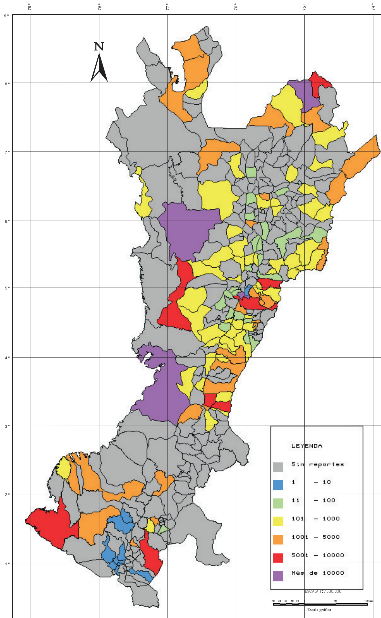
Fig. 32. Personas afectadas por desastres
